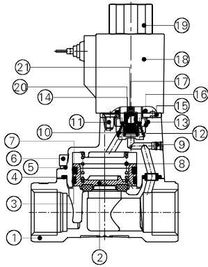
2KLA150出線式
