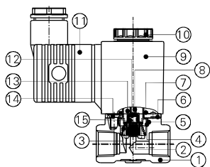
2KLA030DIN插座式
