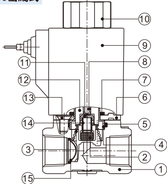
2KWA030出綫式
