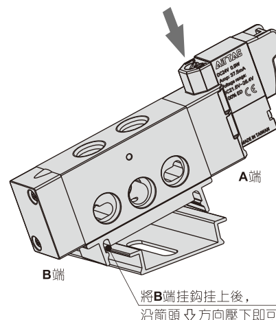
圖1：安裝電磁閥方法
