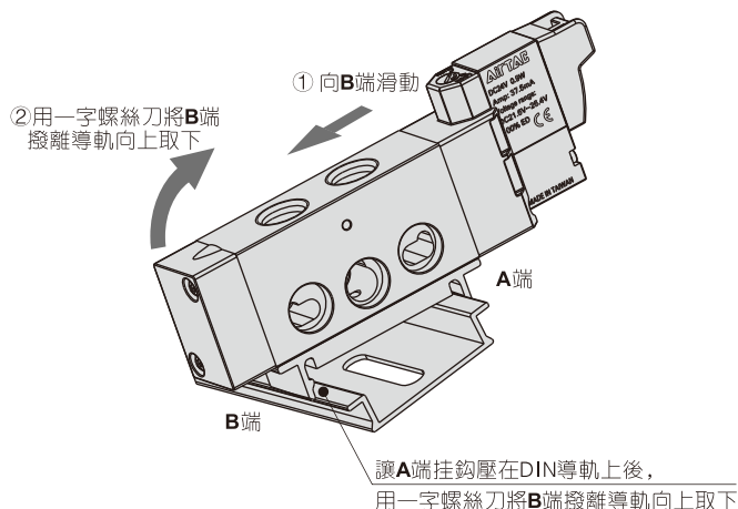
圖2：拆下電磁閥方法
