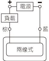
1、一般接線方式
