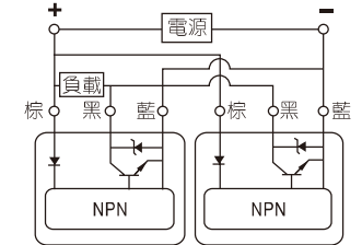
3、并聯接線方式
