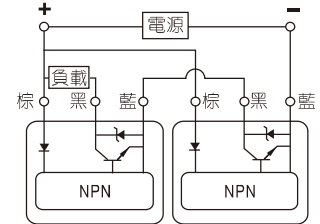
2、串聯接線方式
