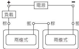
2、串聯接線方式
