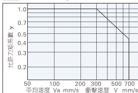
圖綫2 允許力矩系數：γ
