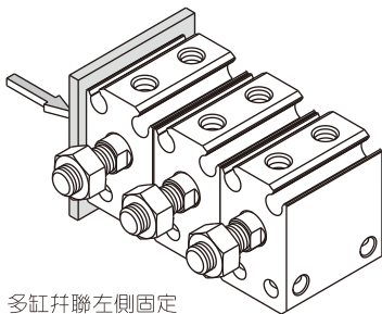
多缸并聯左側固定
