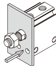
軸向前端固定
