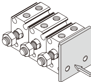
多缸并聯右側固定
